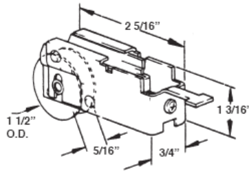
#535 PATIO DOOR ROLLER
