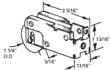
#539 PATIO DOOR ROLLER
