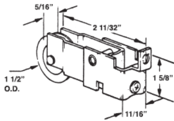
#594 PATIO DOOR ROLLER
