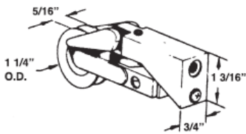
#598 PATIO DOOR ROLLER
