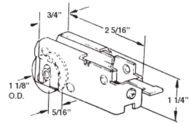
#529 PATIO DOOR ROLLER
