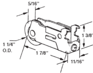
#528 PATIO DOOR ROLLER
