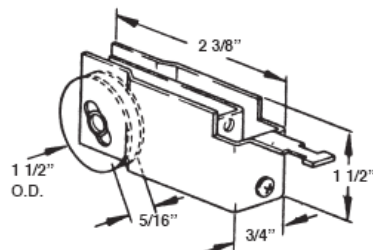
#525 PATIO DOOR ROLLER
