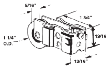
#599 PATIO DOOR ROLLER
