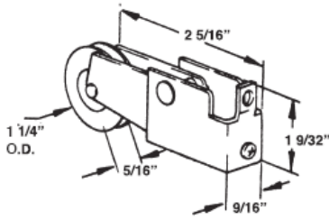
#593 PATIO DOOR ROLLER
