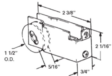
#523 PATIO DOOR ROLLER
