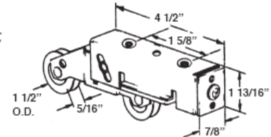
#540 PATIO DOOR ROLLER
