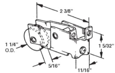
#520 PATIO DOOR ROLLER
