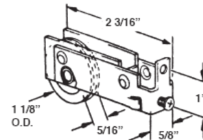
#536 PATIO DOOR ROLLER
