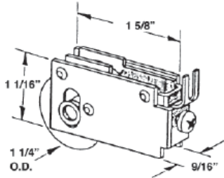
#513 CROSSLY PATIO DOOR ROLLER
