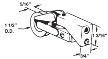
#597 PATIO DOOR ROLLER
