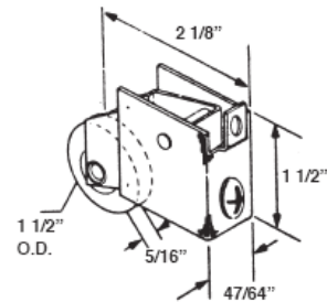
#533 PATIO DOOR ROLLER
