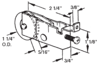
#530 PATIO DOOR ROLLER
