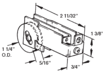
#524 PATIO DOOR ROLLER
