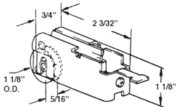
#530 PATIO DOOR ROLLER
