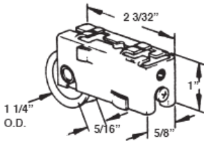
#534 PATIO DOOR ROLLER
