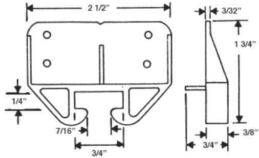
#416 DOOR TRACK SLIDE GUIDE
