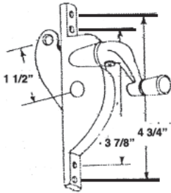
#788 D-7 R.H. JTW OPERATOR
