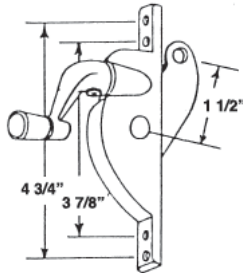
#789 D-7 L.H. JTW OPERATOR
