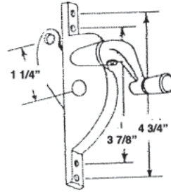
#786 LUDMAN OPERATOR R.H.
