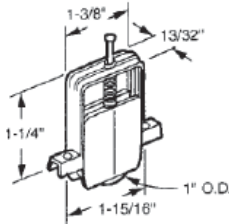
#685 SCREEN DOOR ROLLER
