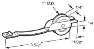
#675 COLUMBIA - UNI-FIT SCREEN DOOR ROLLER
