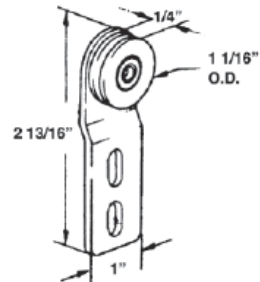
#669 PREMIER SCREEN DOOR ROLLER ASSY
