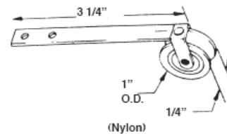
#632 SCREEN DOOR ROLLER
